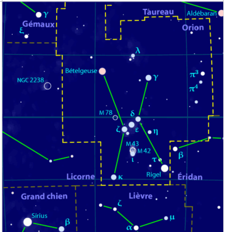
Orion
