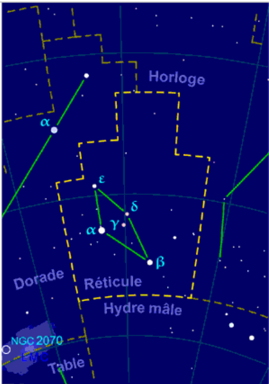
Réticule
