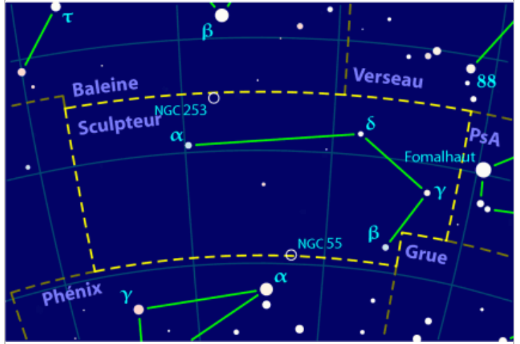
Sculpteur
