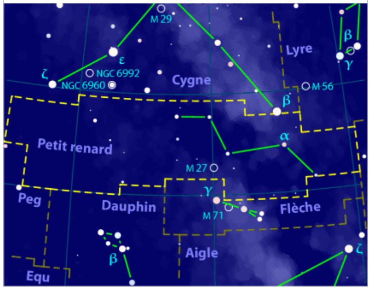
Petit Renard
