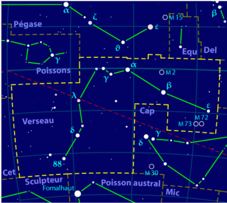
Verseau
