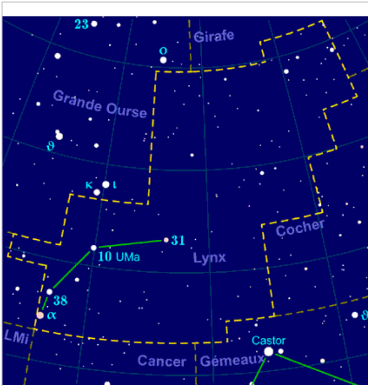
Lynx
