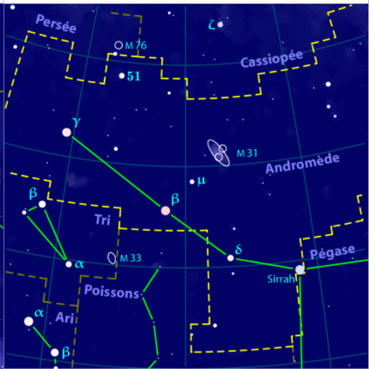
Andromède
