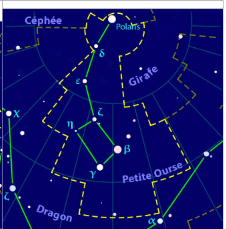
Petite Ourse
