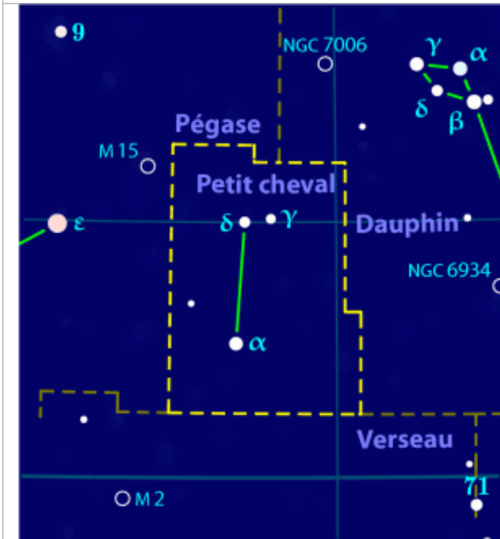
Petit Cheval
