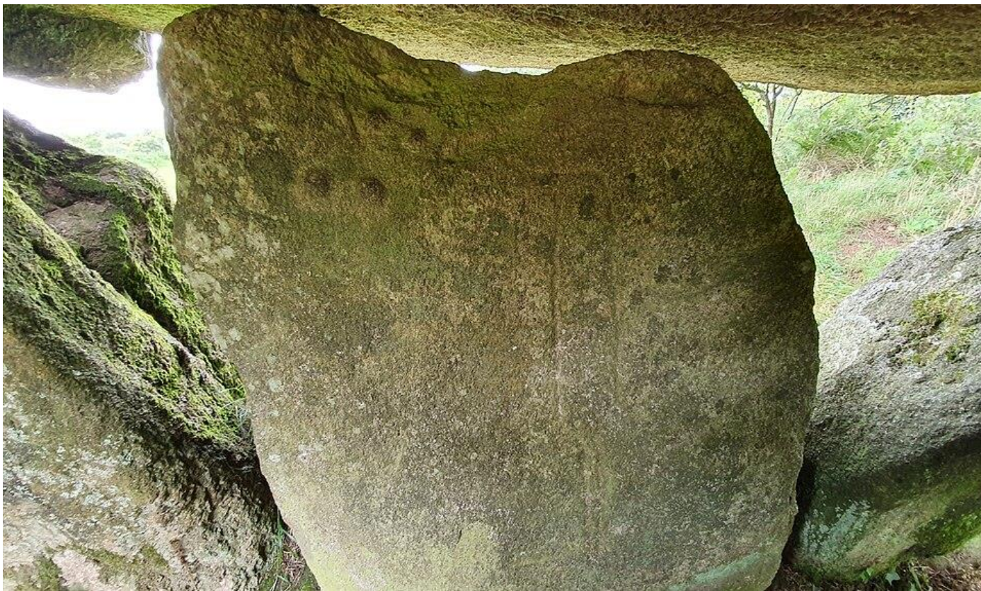
Figuration de la «déesse mère» et de la «palette»
